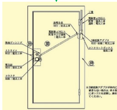
<電気錠扉※>
